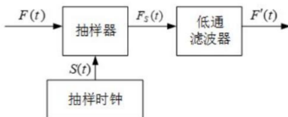
图 2: 信号自然抽样及恢复实验流程图
